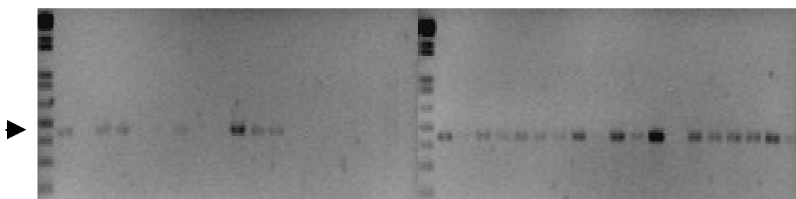
Figura 1. Amplificação do fragmento de 533pb correspondente ao gene mecA em 25 espécimes de estafilococos com resistência a oxacilina isolados de mastites recorrentes de oito propriedades rurais da região de Uberlândia-MG.
