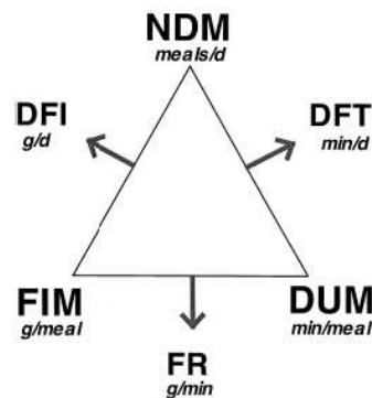
Figura 2: Componentes do comportamento ingestivo e suas interrelações. NDM = número de refeições diárias, FIM = média da ingestão de alimentos por refeição, DUM = média da duração das refeições, DFI = ingestão diária de alimentos, DFT = tempo diário em alimentação, FR = frequência de alimentação.
