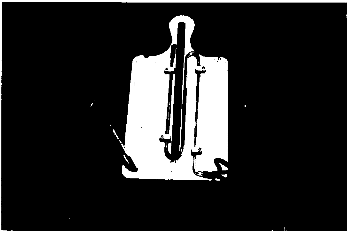
* 1 - Manômetro usado no experimento piloto. Leitura em coluna de Mercúrio, graduada em mm-Hg.
