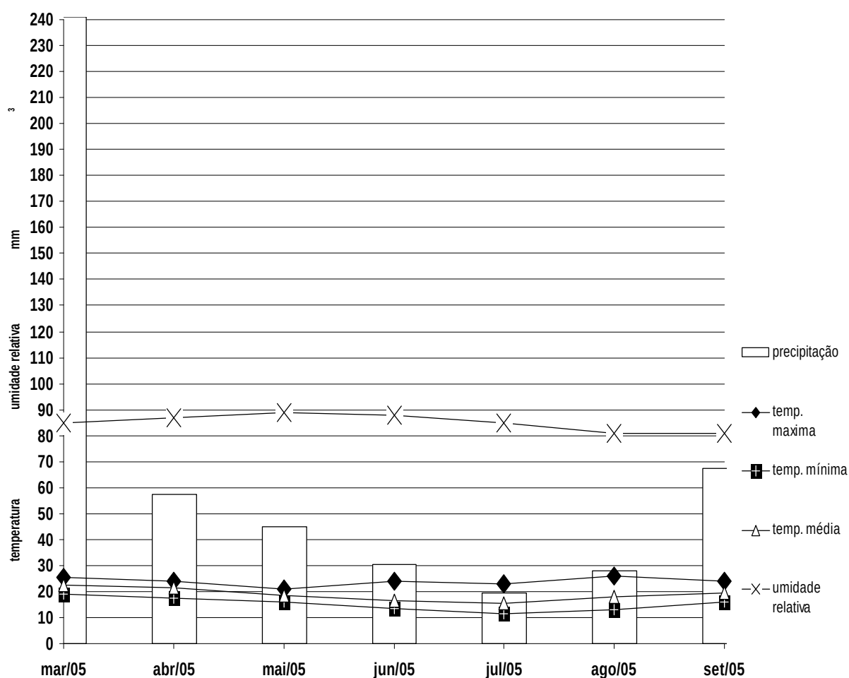
Gráfico 10 – Temperatura média mensal; mínima, média e máxima, umidade relativa do ar (%) e precipitação pluvial total mensal (mm 3 ) registradas no período de março a setembro de 2005, em Viçosa, Minas Gerais.
