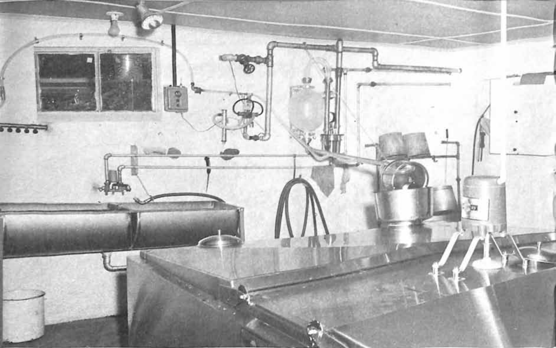
Aparelhos instalados em uma sala da leiteria: válvulas para lavar simultaneamente seis mangueiras de ordenhadeiras mecânicas, lavador de água quente e fria, controle elétrico de todo o sistema de ordenha, tanque de refrigeração em aço inoxidável.
