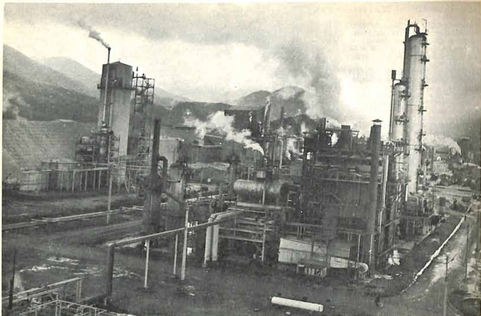
Fábrica de Amônia — é o núcleo principal do Complexo Industrial de Fertilizantes da Ultrafertil.
